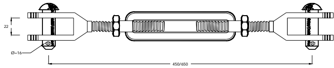
ALZADO
